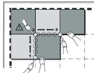
Fig. 4 Méthode de pose des dalles INVISIBLE, BUSINESS
