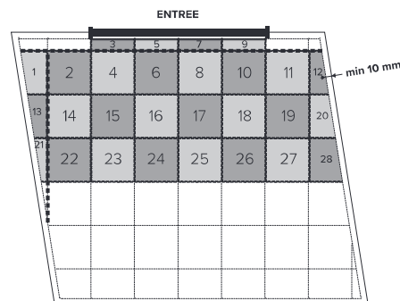
Fig. 3 Sens de pose des dalles INVISIBLE, BUSINESS
